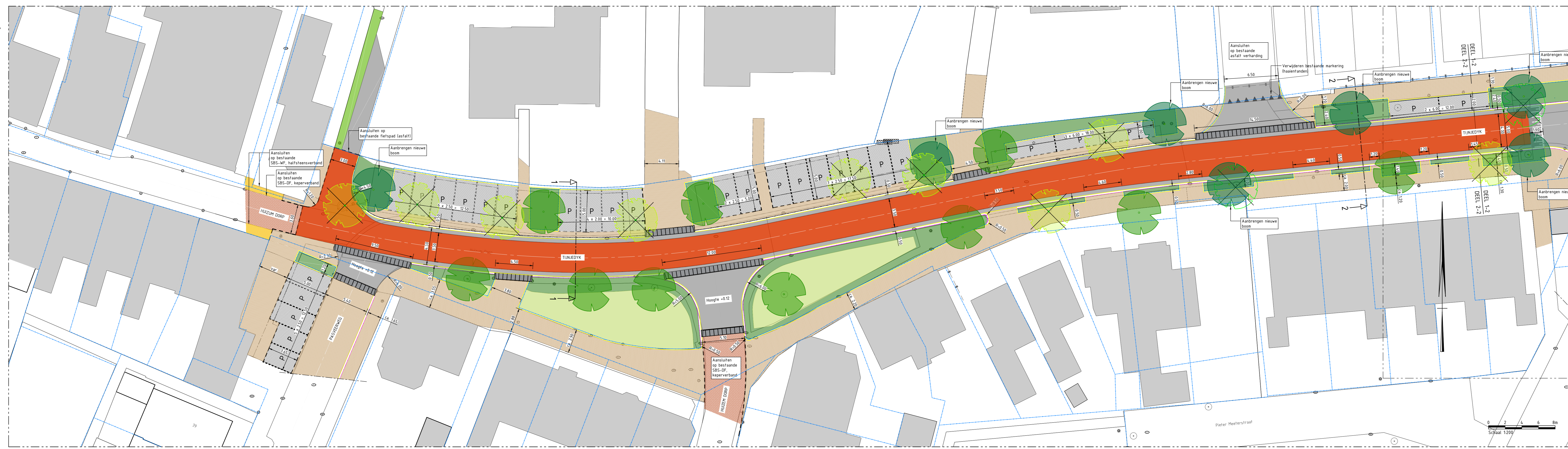
Situatie 2 - 2 1: 200
