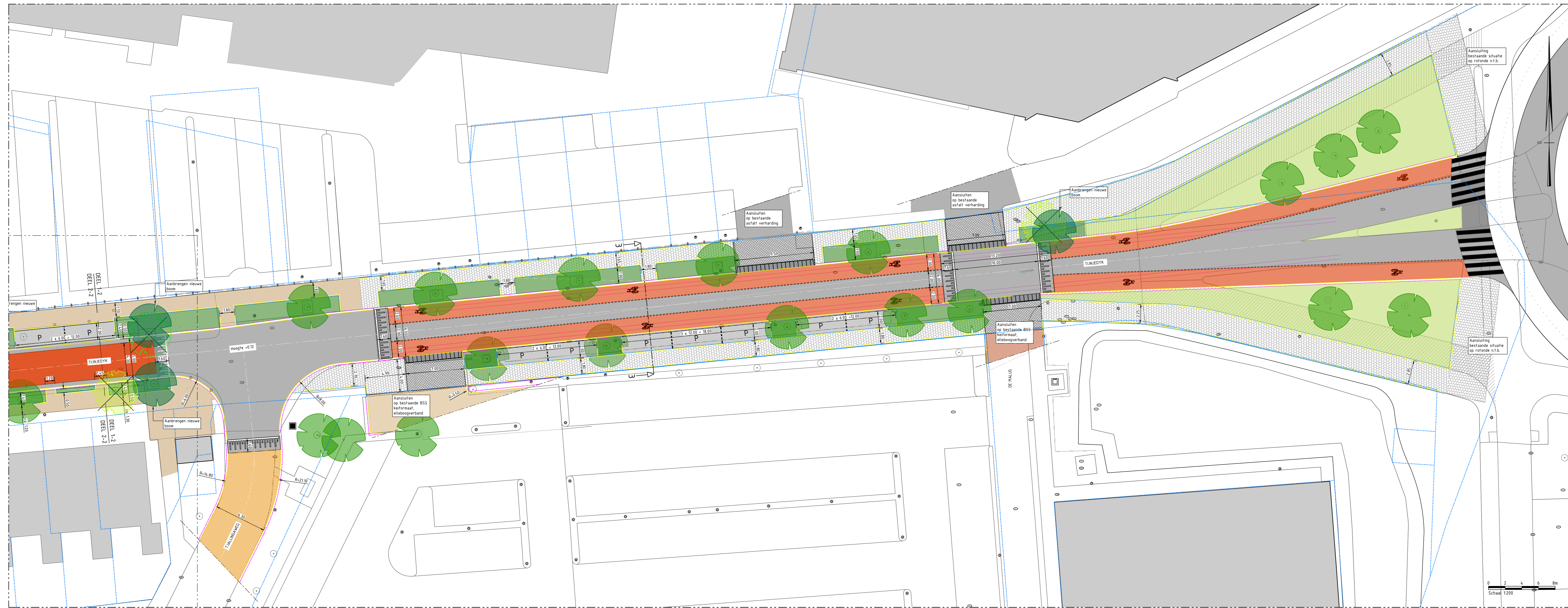
Situatie 1 - 2 1: 200
